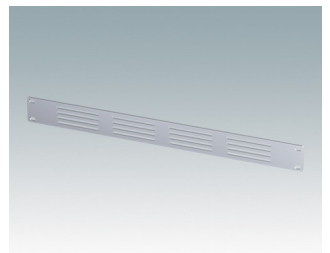
M6019011 Frontplatte 1HEx19" mit Lüftung Aluminium Matt eloxiert 482,6x3x43,6mm
